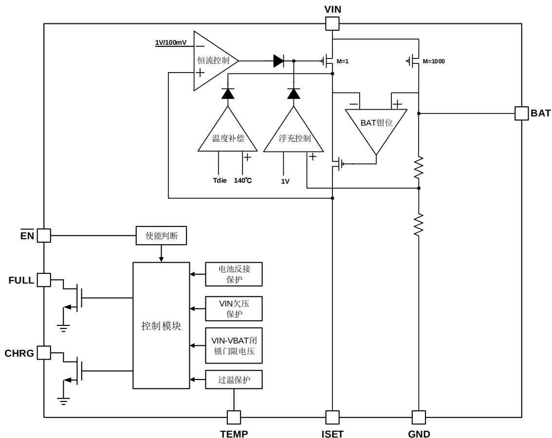
图 1. GD30BC1503 功能框图
