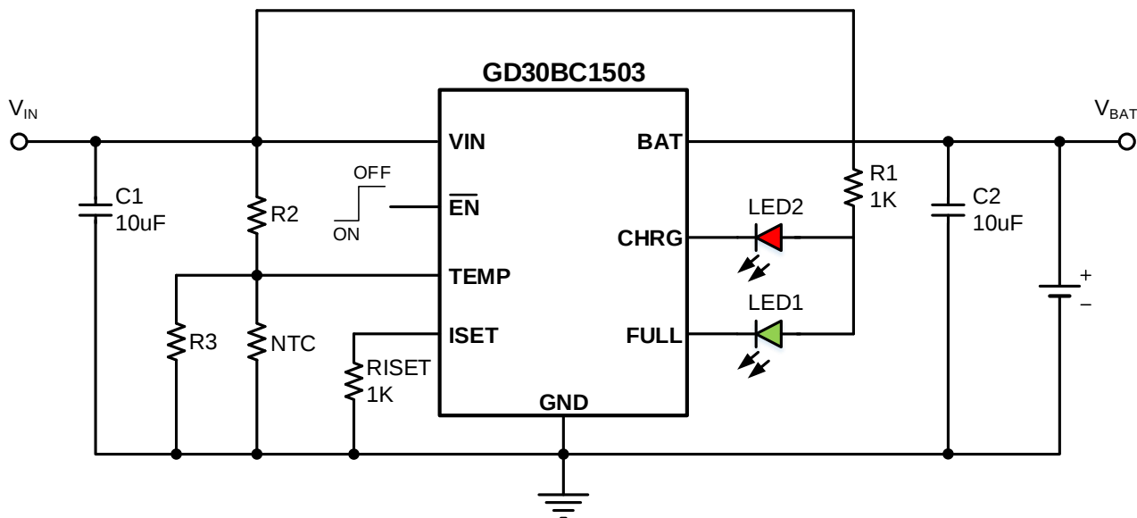
图 3. 1A 恒流充电参考电路
